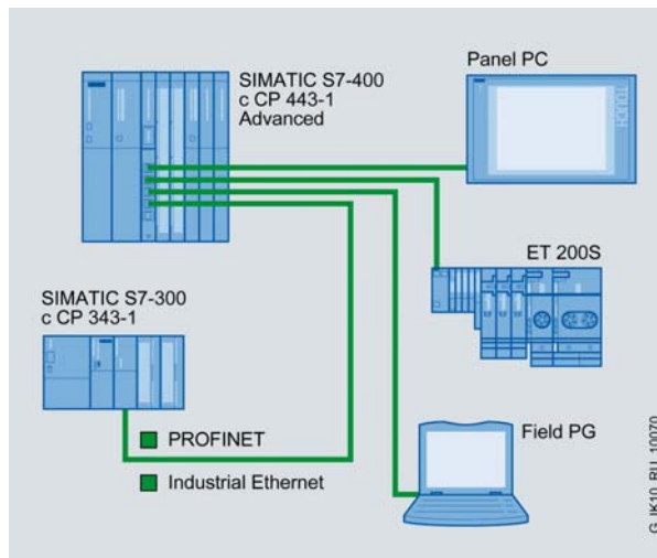
Небольшая локальная сеть PROFINET на основе коммуникационного процессора CP 443-1 Advanced
