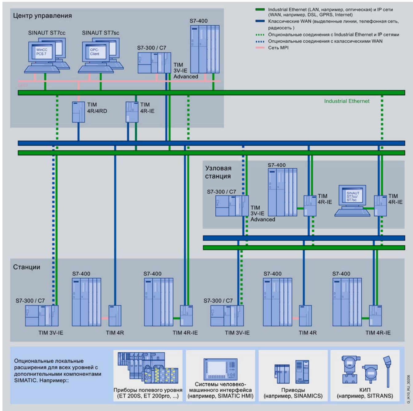
Система телеуправления SINAUT ST7
