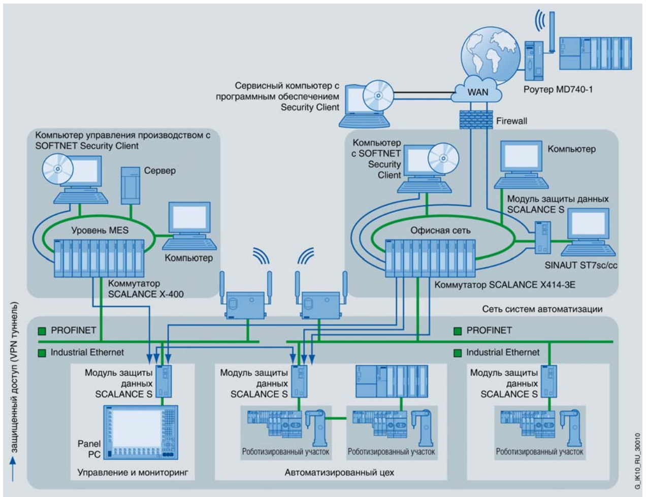
Защита данных с помощью модулей SCALANCE S
