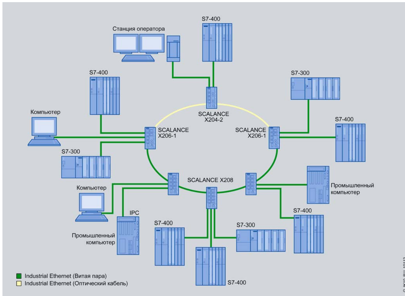
Конфигурация со скоростным реконфигурированием гибридной кольцевой структуры
