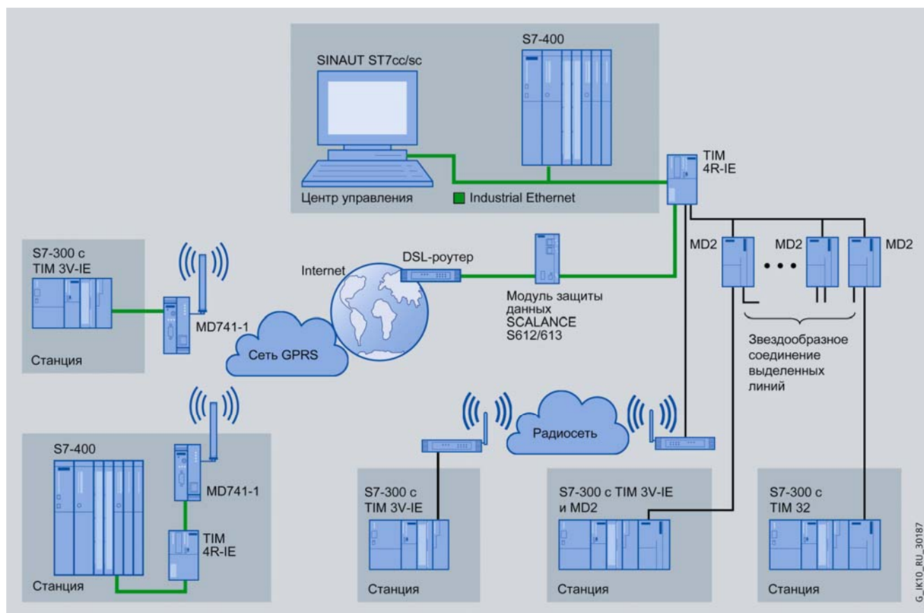
Различные виды каналов связи системы SINAUT ST7
