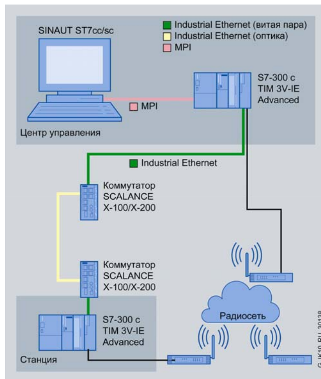
Резервированные соединения компонентов SINAUT ST7 через WAN
