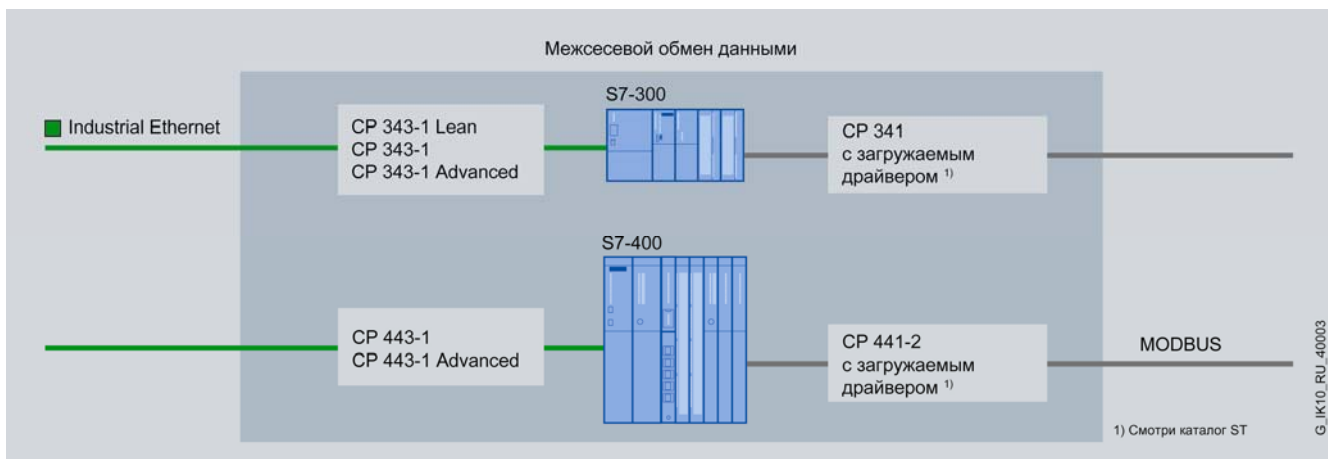
Обмен данными между сетями Industrial Ethernet и MODBUS
