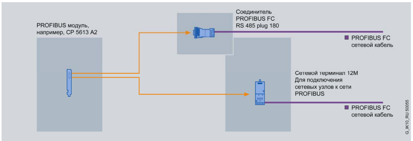
Типовой вариант подключения к электрической (RS 485) сети с помощью соединителя PB FC RS 485 или сетевого терминала
