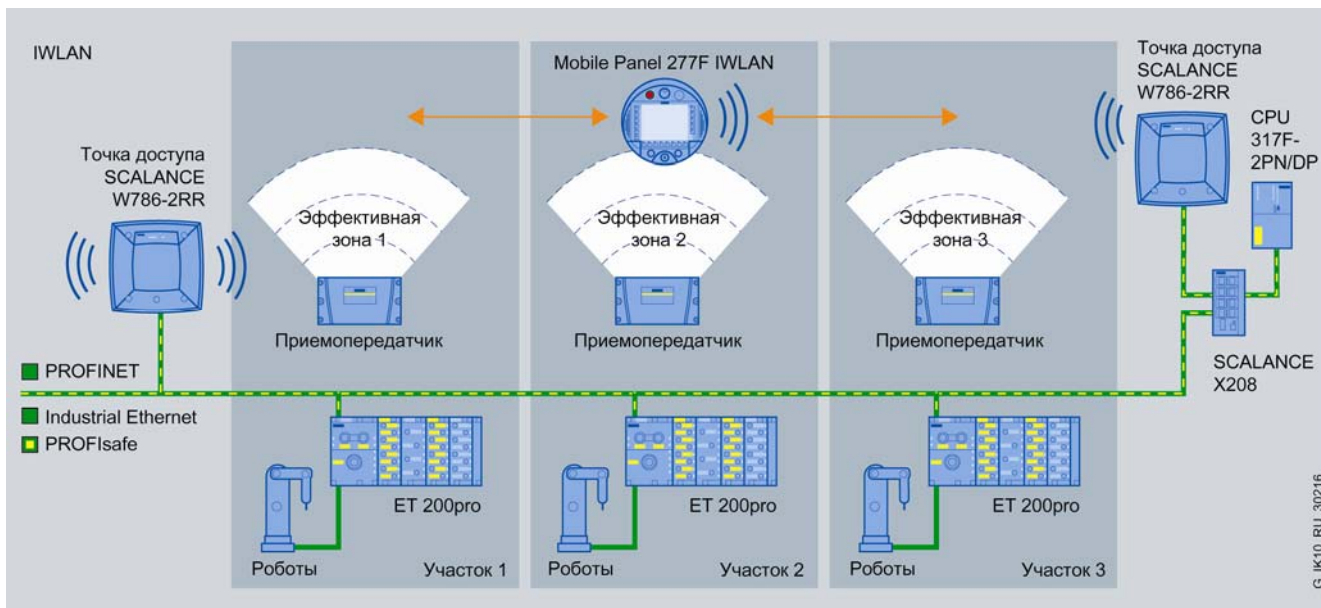
Оперативное управление и мониторинг работы роботов с поддержкой функций обеспечения безопасности.
