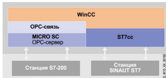
Объединение систем SINAUT MICRO и SINAUT ST7 в компьютерном центре управления на базе WinCC
