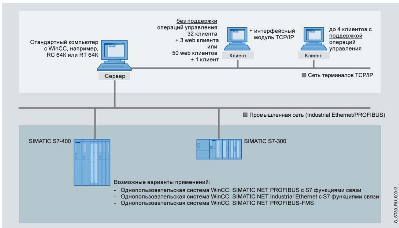
Многопользовательская система WinCC
