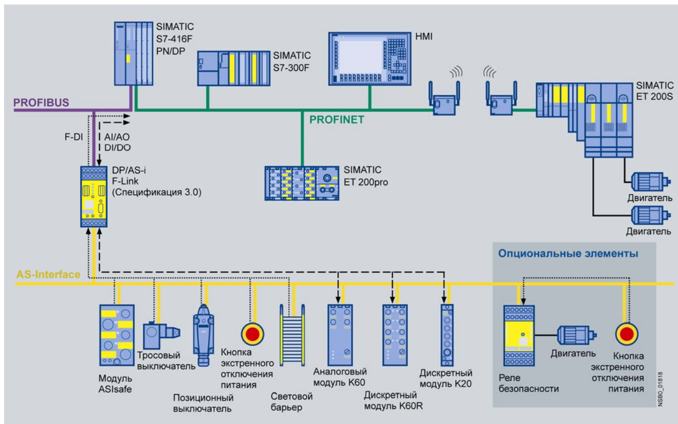
Интеграция приборов ASIsafe в сеть PROFIBUS с F контроллером SIMATIC S7. Вариант 2
