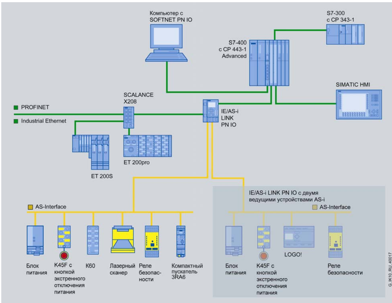
Подключение сети AS-Interface к сети PROFINET через модуль IE/AS-i Link PN IO
