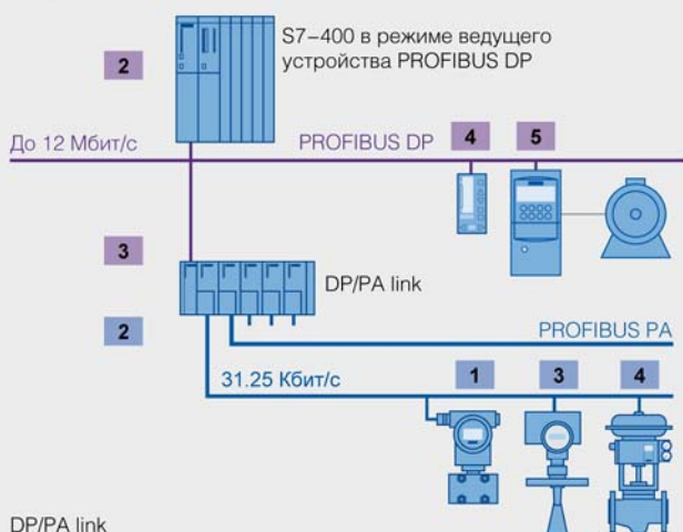
Скоростное решение на базе блока DP/PA link
