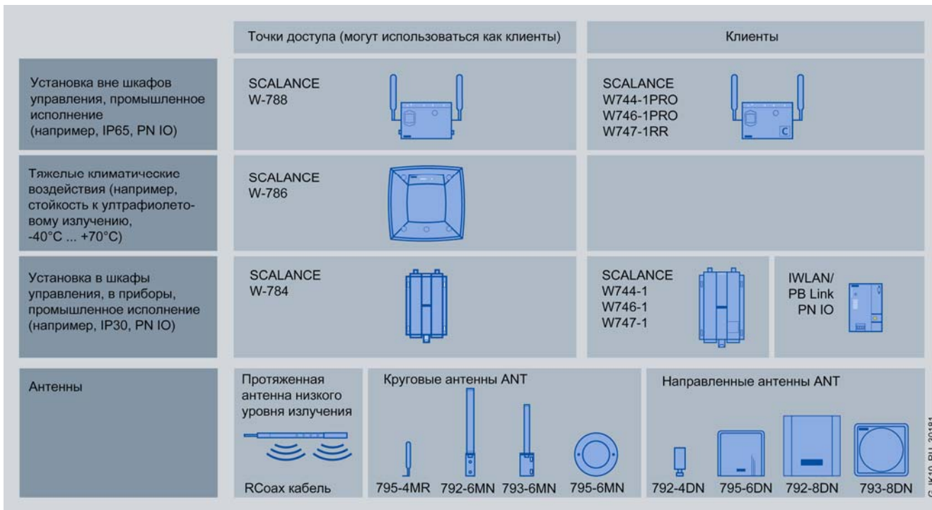
Позиционирование точек доступа и модулей клиентов
