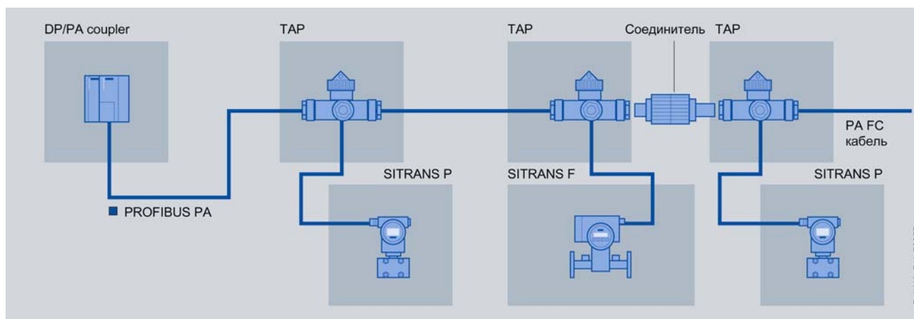
Пример подключения компонентов к сети PROFIBUS PA
