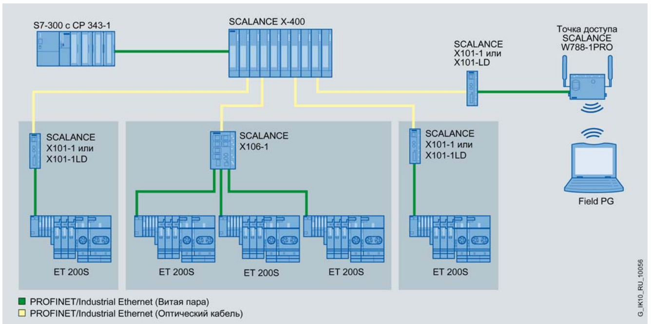
Оптическая звездообразная структура с конверторами SCALANCE X101-1/X101-1LD и удаленной точкой доступа SCALANCE W
