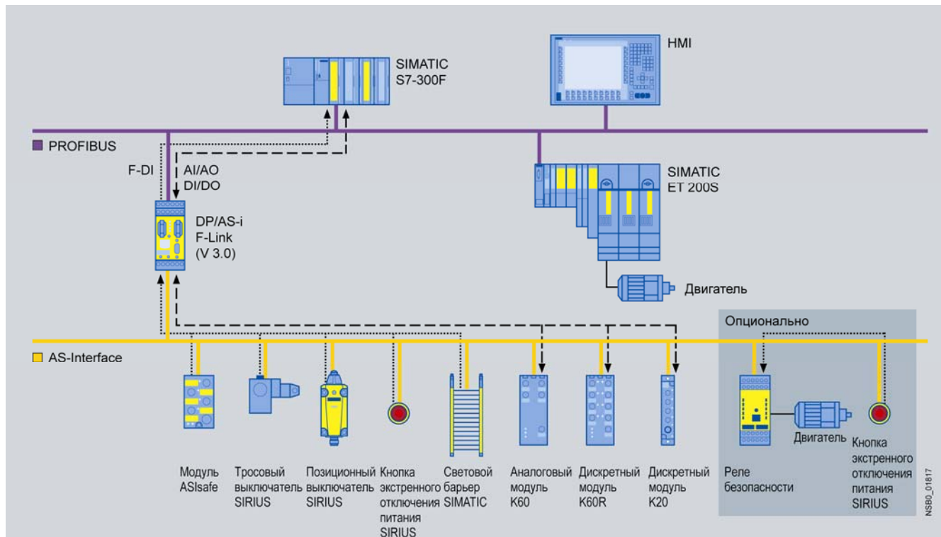
Интеграция приборов ASIsafe в сеть PROFIBUS с F контроллером SIMATIC S7. Вариант 1
