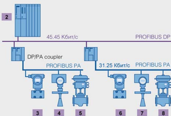
Рентабельное решение с непосредственной адресацией
