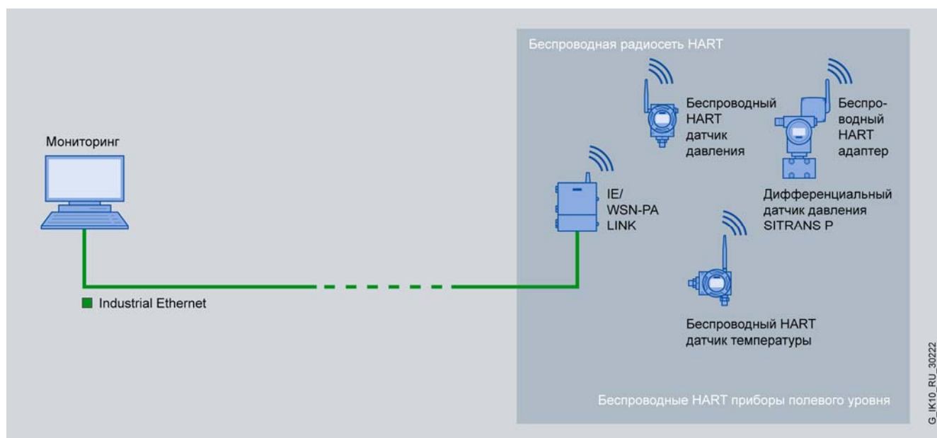
Мониторинг процесса с использованием беспроводного протокола HART
