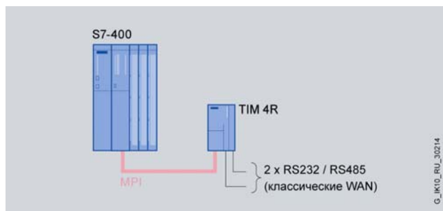
Соединение S7-400 с модулем TIM 4R через MPI
