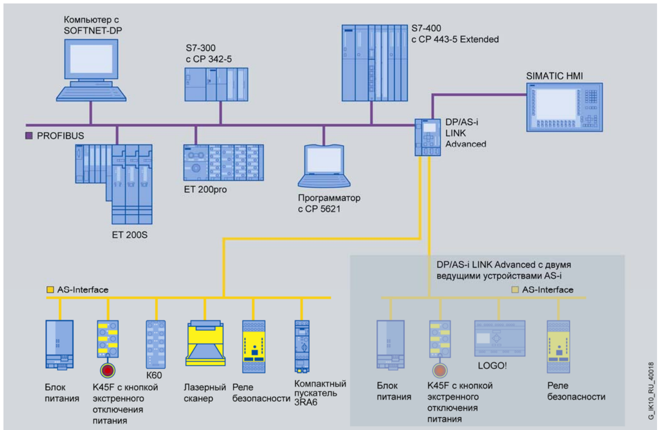
Подключение сети AS-Interface к сети PROFIBUS DP через модуль DP/AS-i Link Advanced
