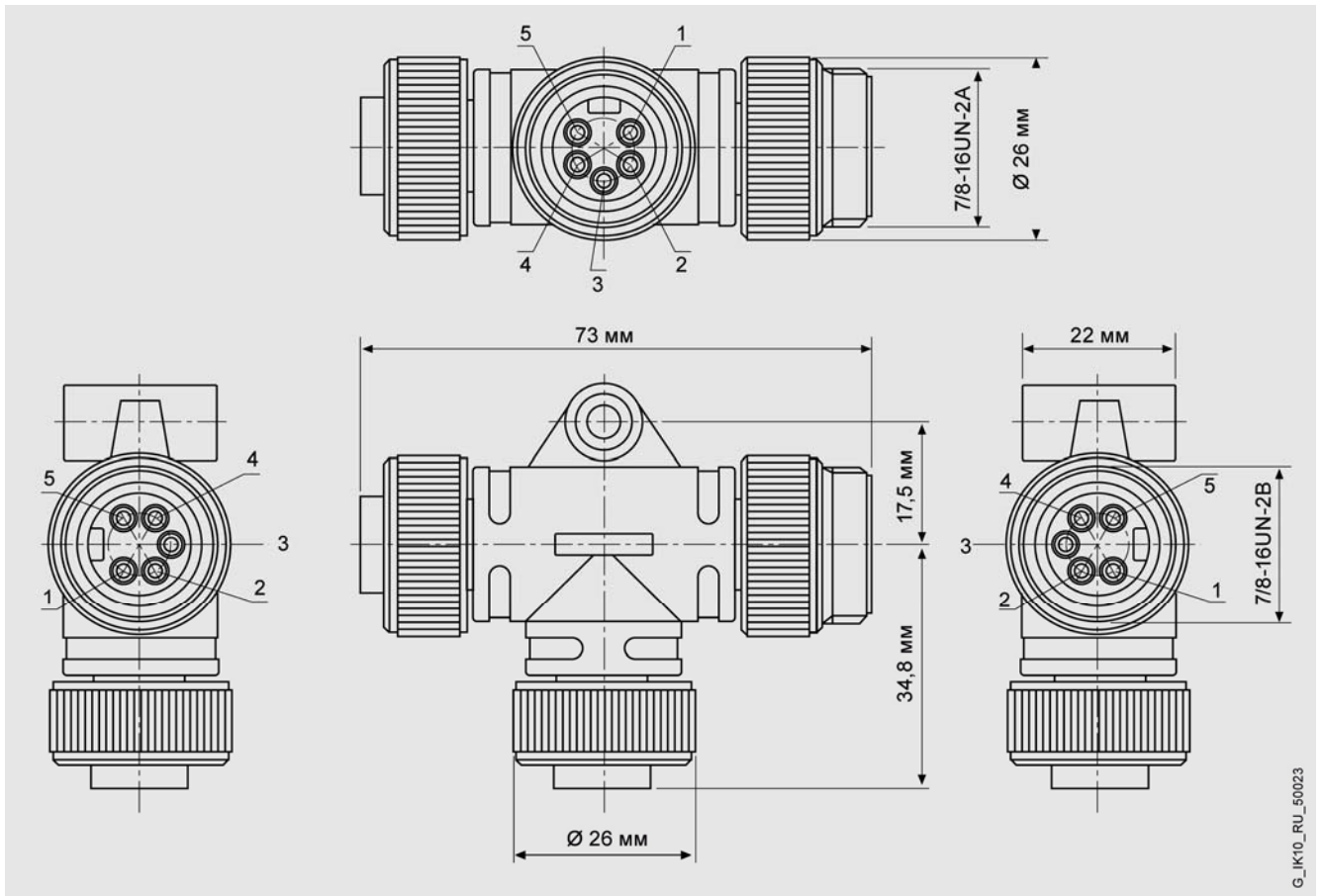
Т-образный соединитель 7/8" T-Tap PRO
