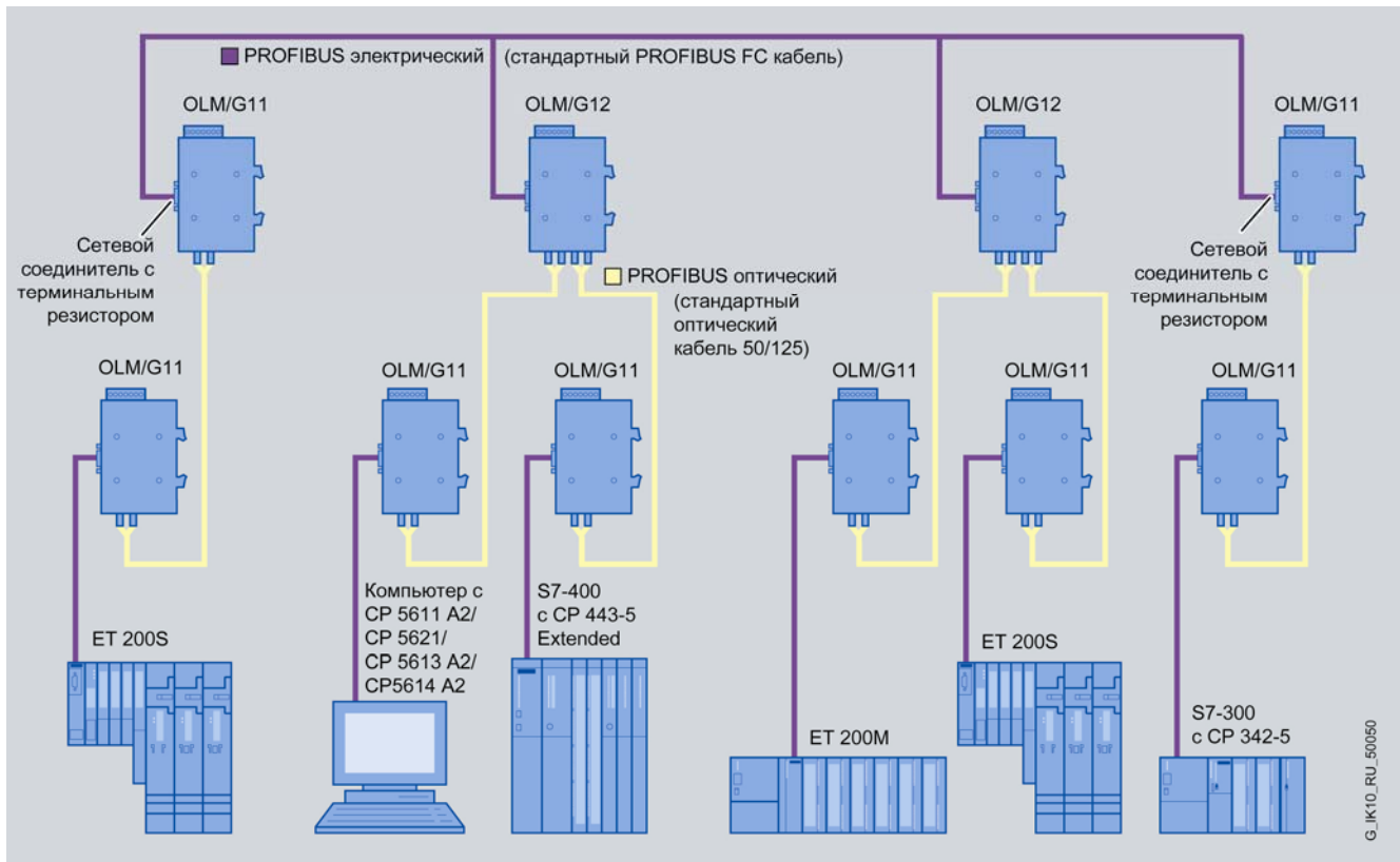
Оптическая звездообразная структура сети PROFIBUS
