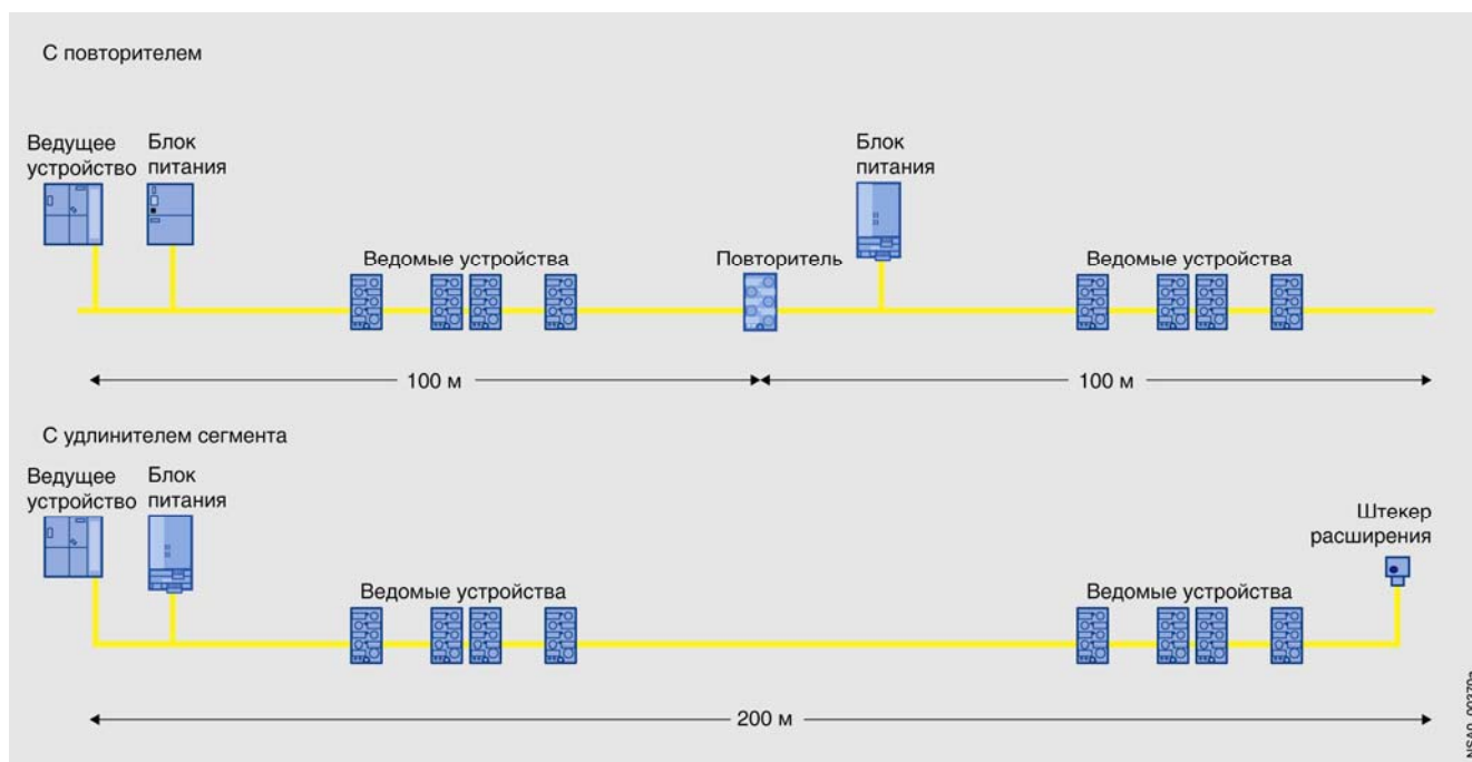
Варианты построения сети AS-Interface протяженностью 200 м
