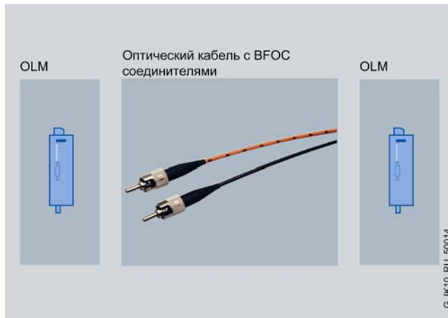
Пример подключения к оптической сети с использованием BFOC соединителей
