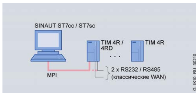
Подключение одного или нескольких модулей TIM 4R к центру управления SINAUT ST7cc/ST7sc через MPI
