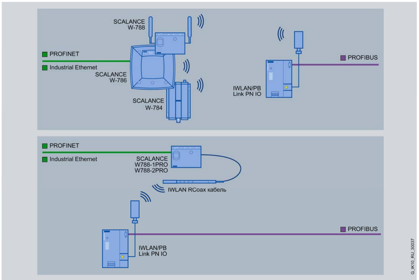
Обмен данными между сетями PROFINET/Industrial Ethernet и PROFIBUS через IWLAN
