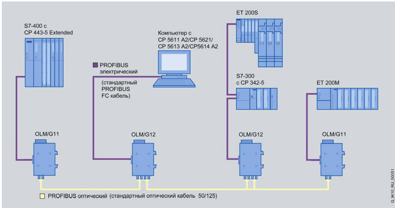
Оптическая магистральная структура сети PROFIBUS
