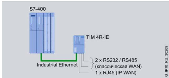
Соединение S7-400 с модулем TIM 4R-IE через Industrial Ethernet
