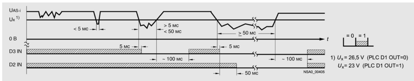
Передача диагностических сигналов штекером расширения исполнения Plus.
