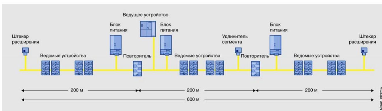
Максимальная конфигурация сети AS-Interface (ведущее устройство подключено к центру сети)
