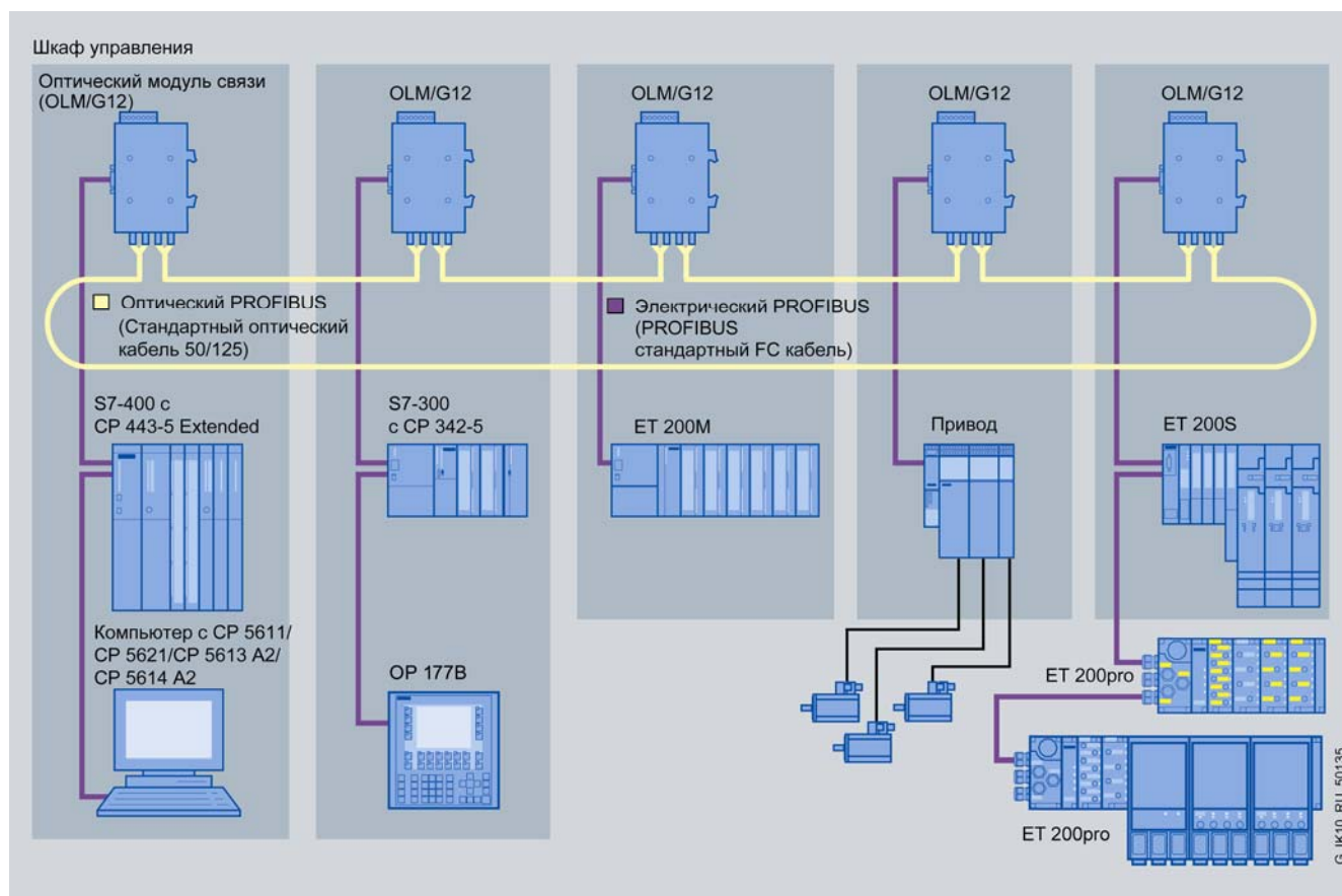
Пример оптической кольцевой структуры сети PROFIBUS на основе модулей OLM
