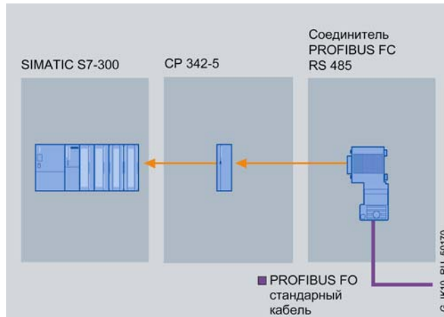
Типовой вариант подключения к электрической (RS 485) сети с помощью соединителя PB FC RS 485
