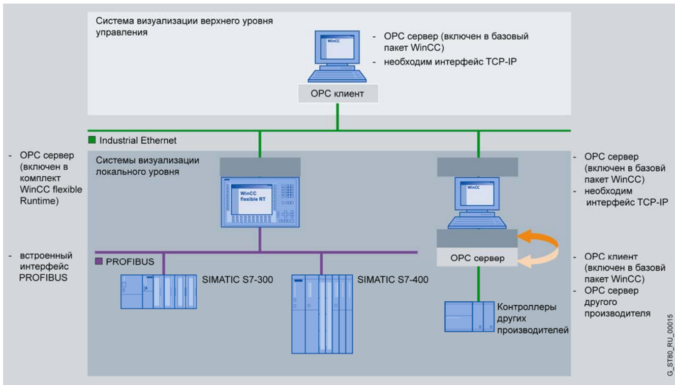
Обмен данными через OPC
