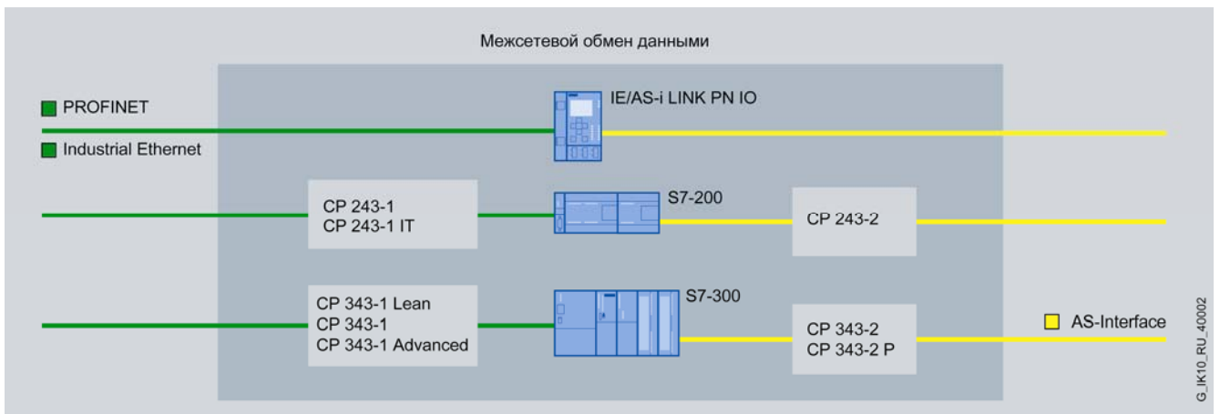
Обмен данными между сетями PROFINET/Industrial Ethernet и AS-Interface
