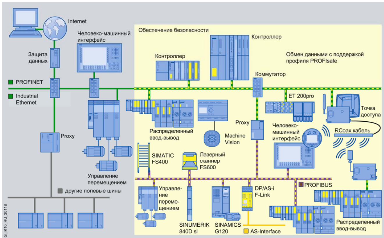
Беспроводной обмен данными с поддержкой профиля PROFISafe
