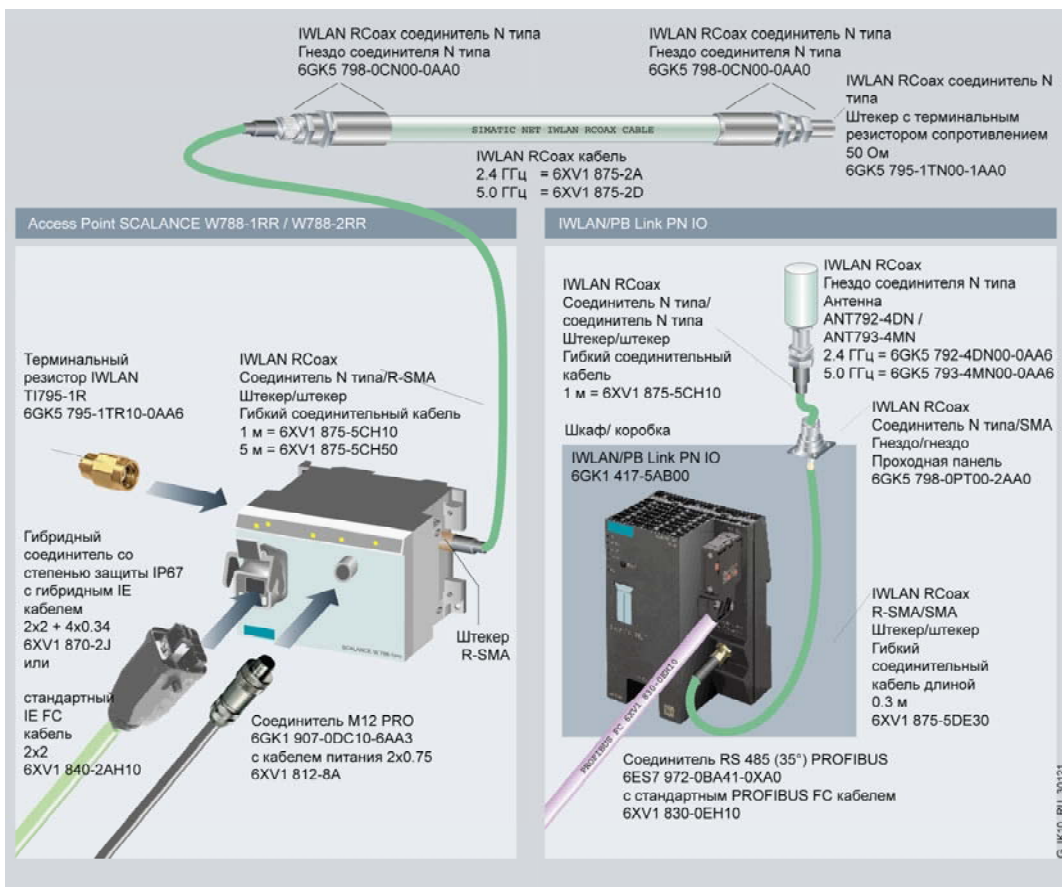
Беспроводное подключение мобильной станции PROFIBUS
