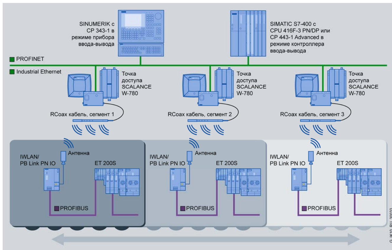
Использование модуля IWLAN/PB Link PN IO в системах управления монорельсовыми системами
