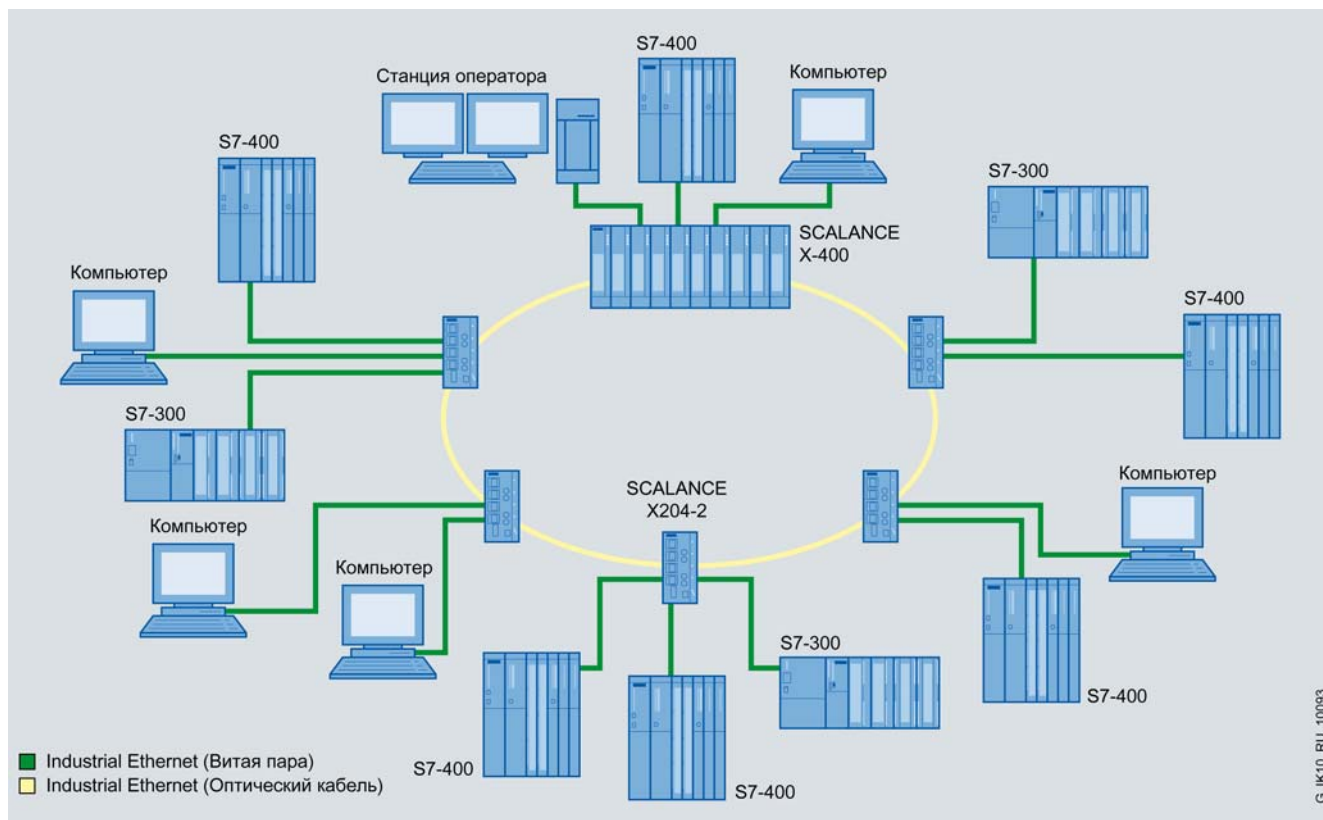
Конфигурация со скоростным реконфигурированием оптического кольца
