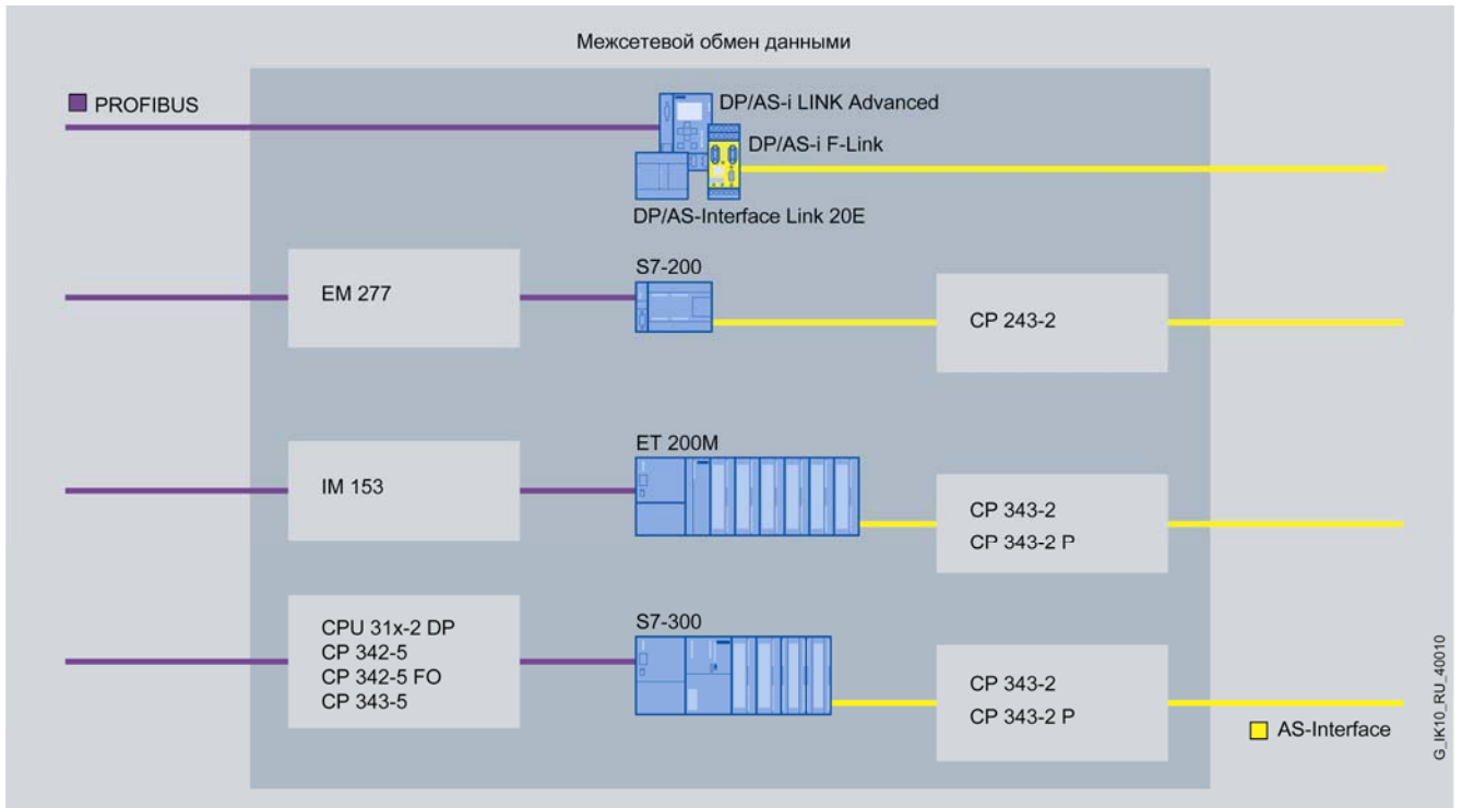
Обмен данными между сетями PROFIBUS и AS-Interface
