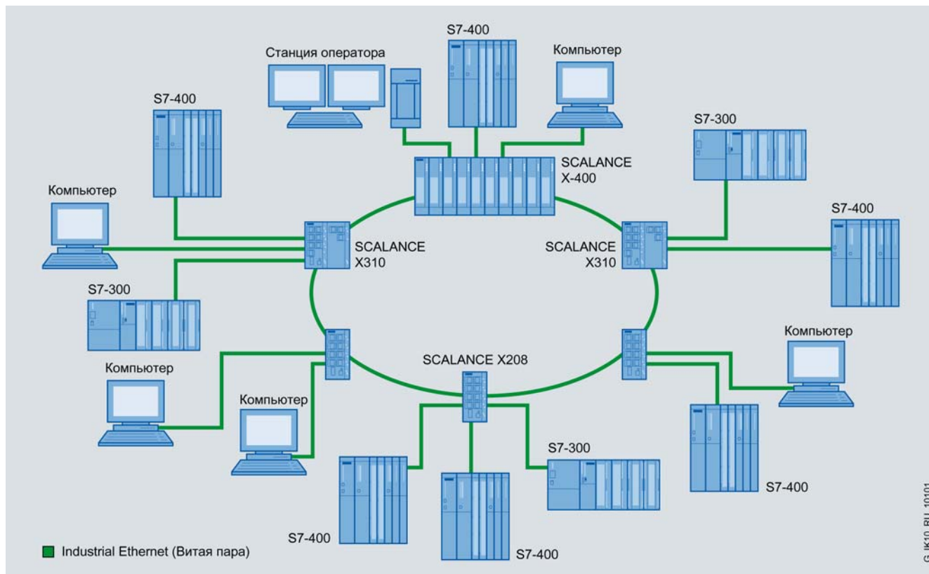
Конфигурация со скоростным реконфигурированием электрического кольца
