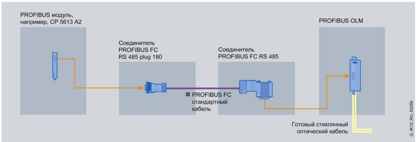
Пример подключения к оптической сети
