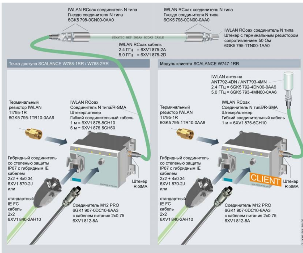
Беспроводное подключение мобильной станции Industrial Ethernet
