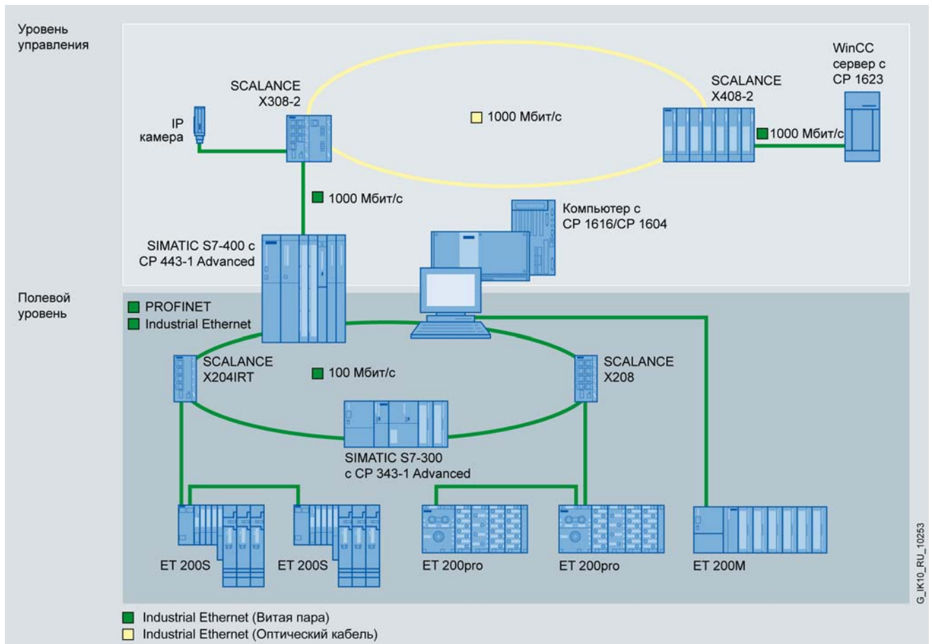
PROFINET IO на основе кольцевых топологий с поддержкой функций реконфигурирования сети (MRP)
