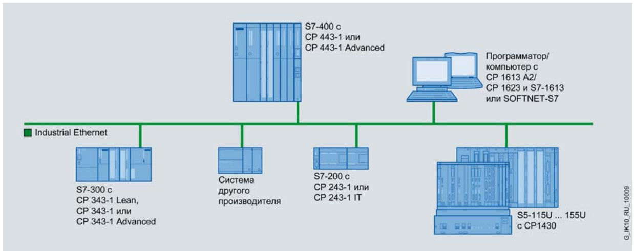
Открытый обмен данными через Industrial Ethernet
