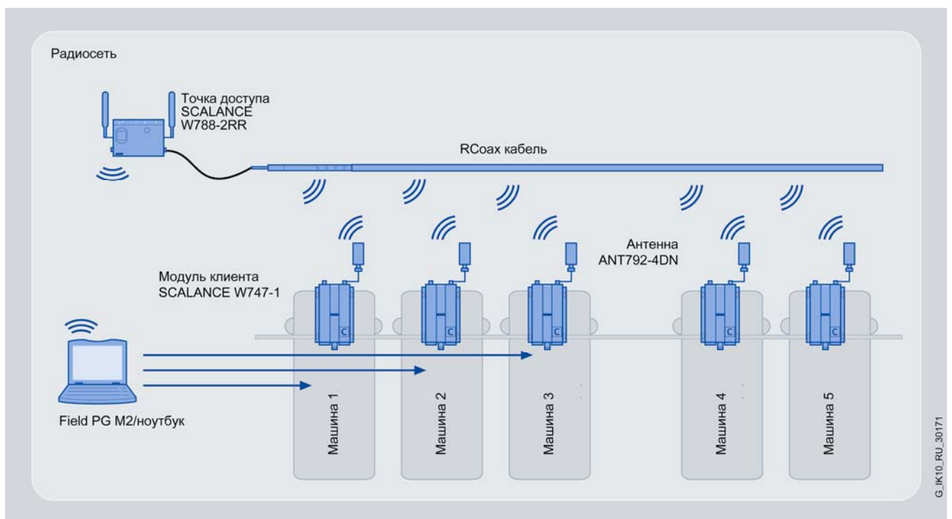
Использование IWLAN для управления монорельсовым конвейером
