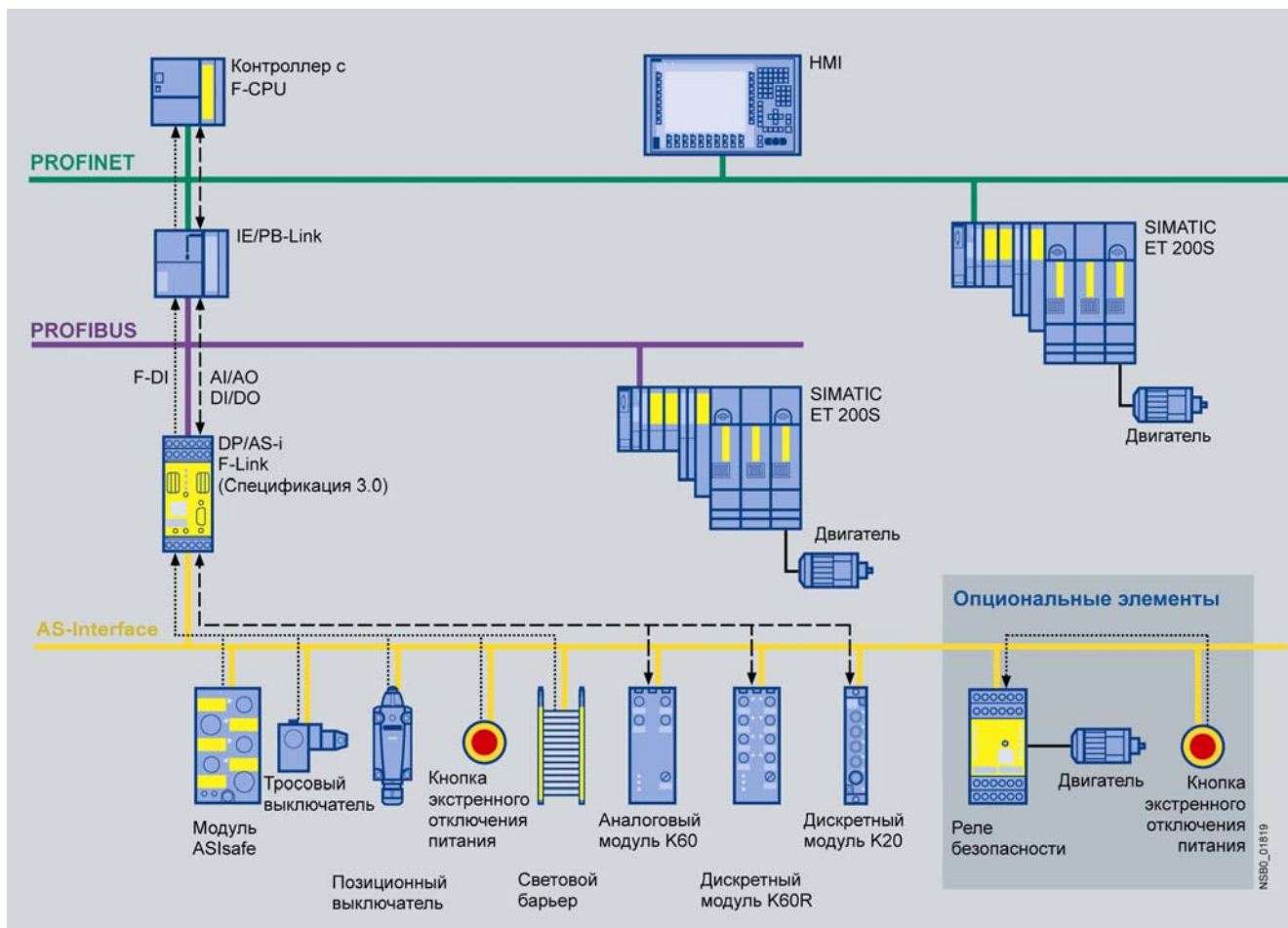
Интеграция приборов ASiSafe в сеть PROFINET с F контроллером SIMATIC S7 через модуль IE/PB Link PN IO
