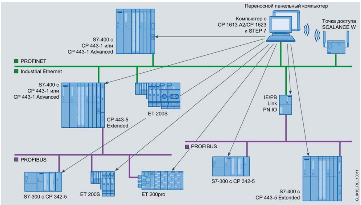
PG/OP функции связи для дистанционного программирования и диагностики всех сетевых станций SIMATIC
