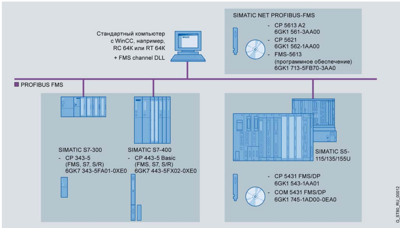
Однопользовательская система WinCC: PROFIBUS FMS
