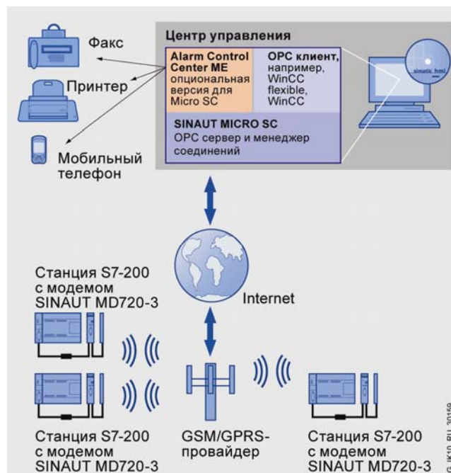
Система телеуправления SINAUT MICRO
