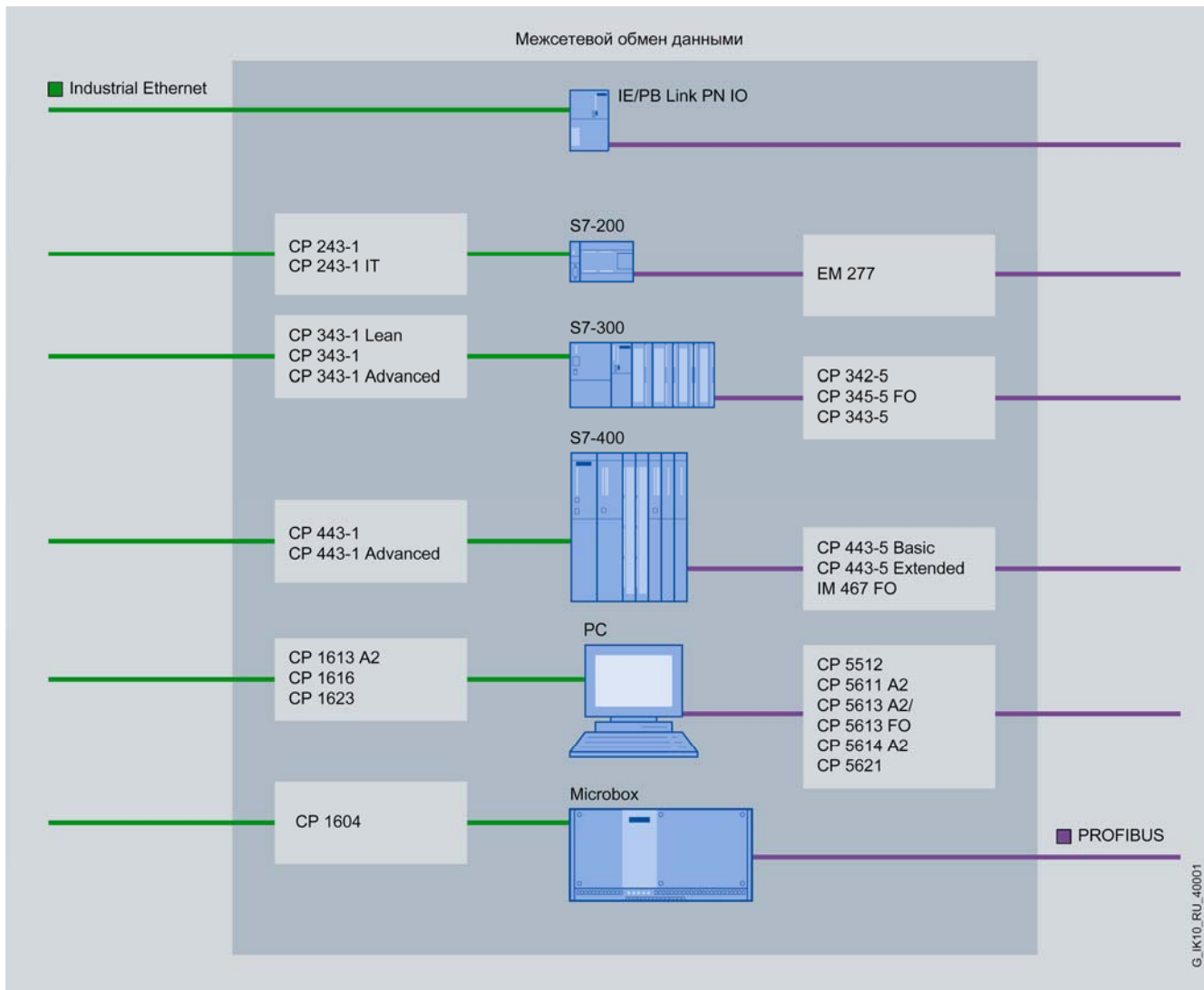
Обмен данными между сетями PROFINET/Industrial Ethernet и PROFIBUS
