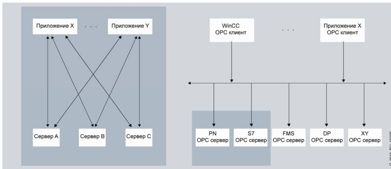
Сравнение клиент/ серверных и OPC архитектур
