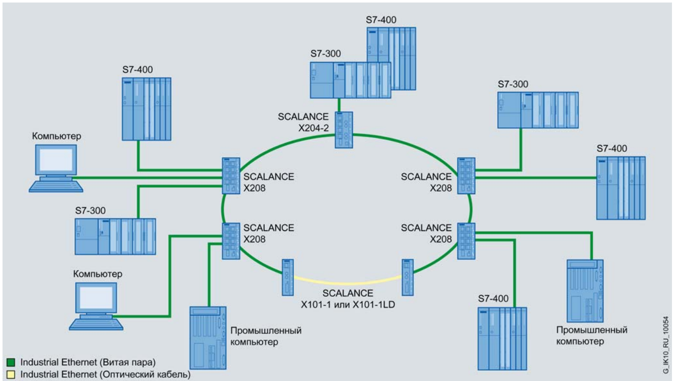
Кольцевая структура с использованием электрических и оптических каналов связи и конверторов SCALANCE X101-1/X101-1LD
