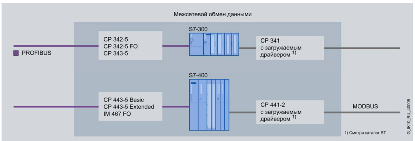
Обмен данными между сетями PROFIBUS и MODBUS
