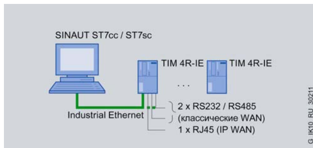
Подключение одного или нескольких модулей TIM 4R-IE к центру управления SINAUT ST7cc/ST7sc через Industrial Ethernet
