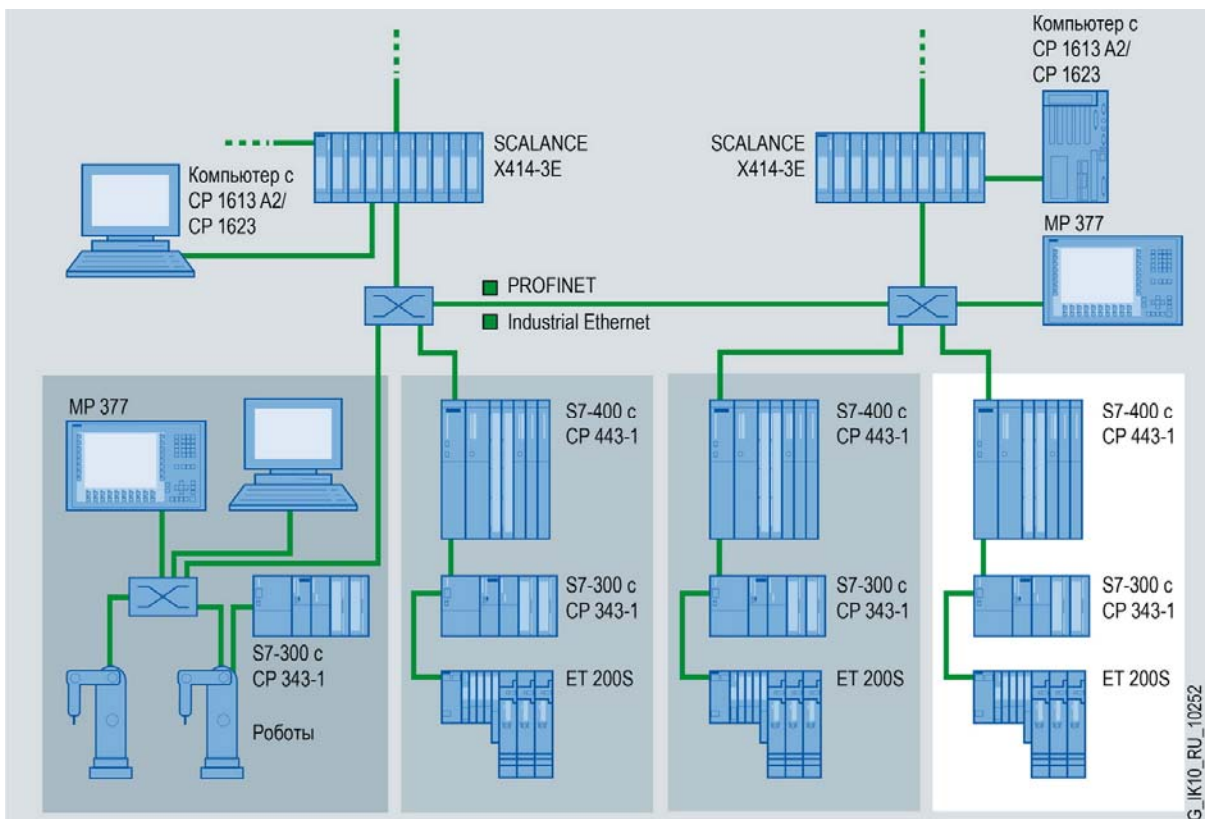
Высокопроизводительное коммутуемое соединение 3-го уровня с поддержкой функций резервированного роутинга (VRRP)
