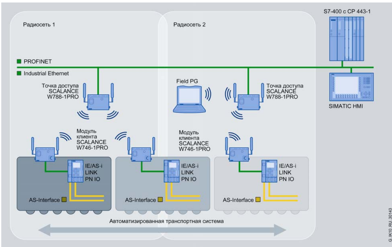
Беспроводный обмен данными между AS-Interface и Industrial Ethernet
