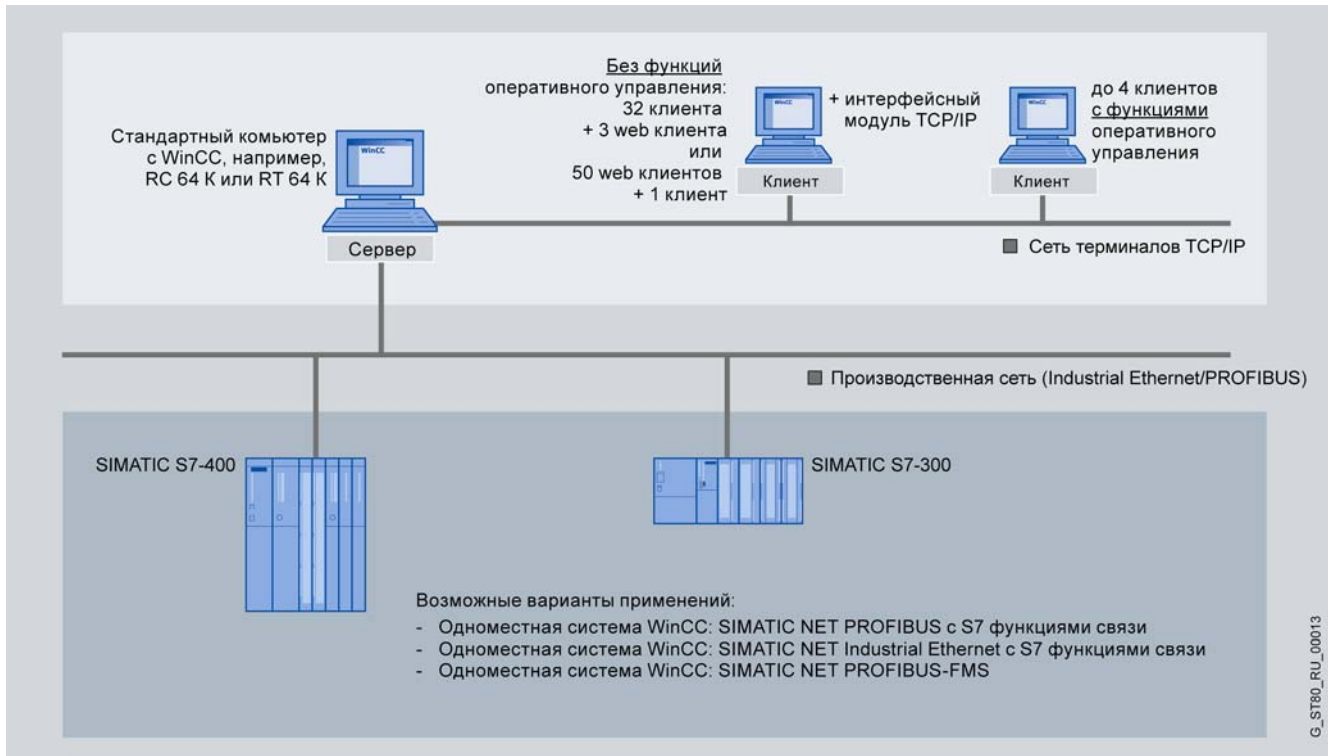
Многопользовательская система SIMATIC WinCC
