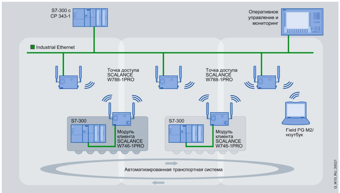
Использование IWLAN для управления работой автоматизированной транспортной системы
